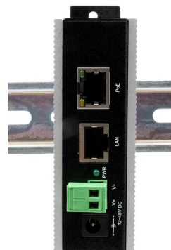
Montage an Tragschiene
