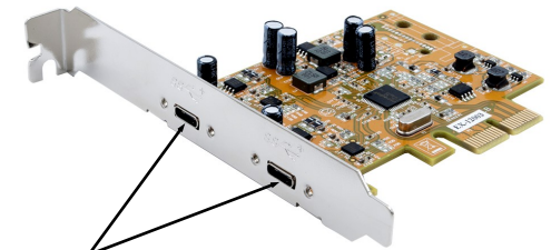
J3 & J4: 2x externe USB 3.2 (Gen2) C-Buchse (verschraubbar)
